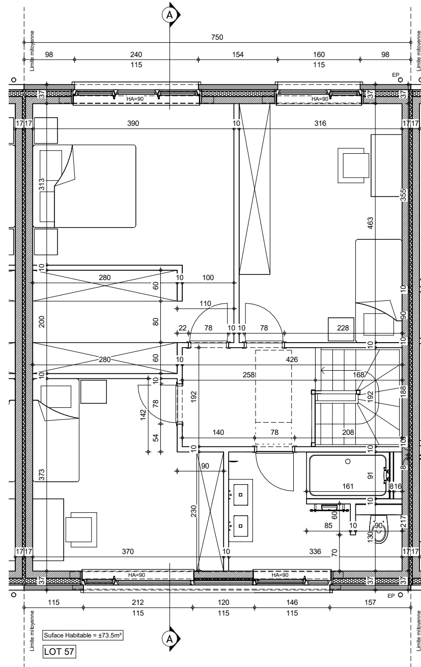
ETAGE
