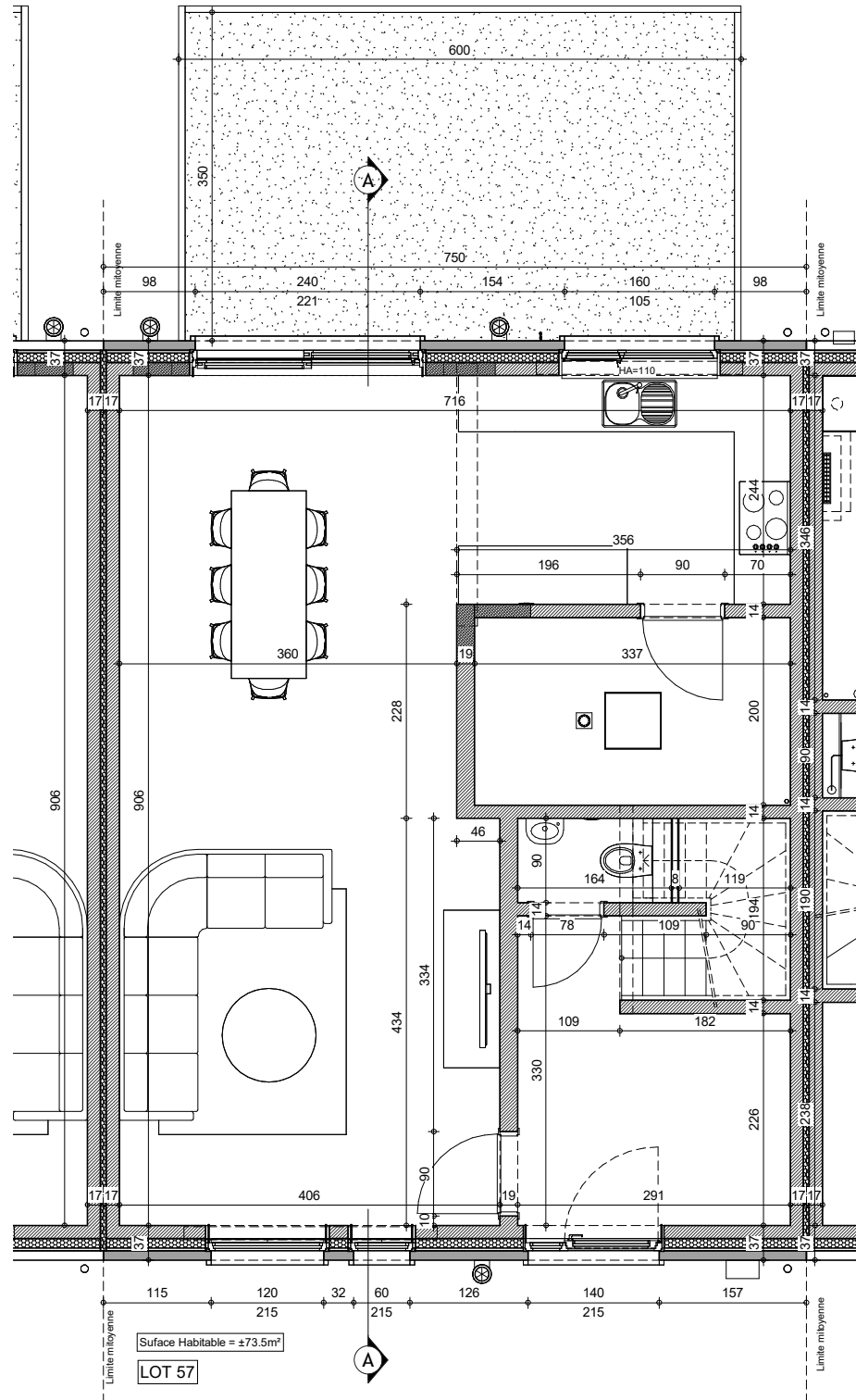
REZ-DE-CHAUSSEE
